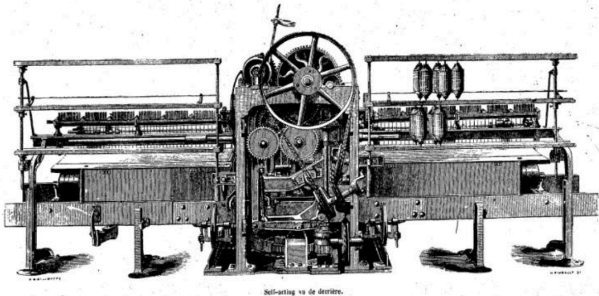
Self-acting, vu de derrière.- Illustration, H. Rimbault, P.-H. Delamotte (TURGAN Julien. Les grandes usines. La Foudre : filature de coton. Tome 3, 1868, p. 173).
