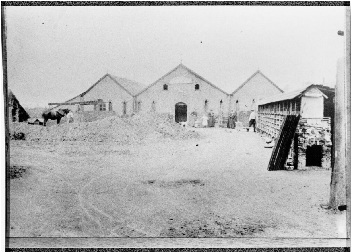
Ateliers de fabrication et cheminée d'usine avant la construction du four à flammes renversées. A gauche et au second plan, malaxeur hippomobile.- Photographie ancienne.
