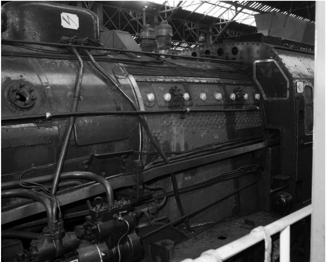
Locomotive, vue latérale, partie droite, détail de la chaudière.
