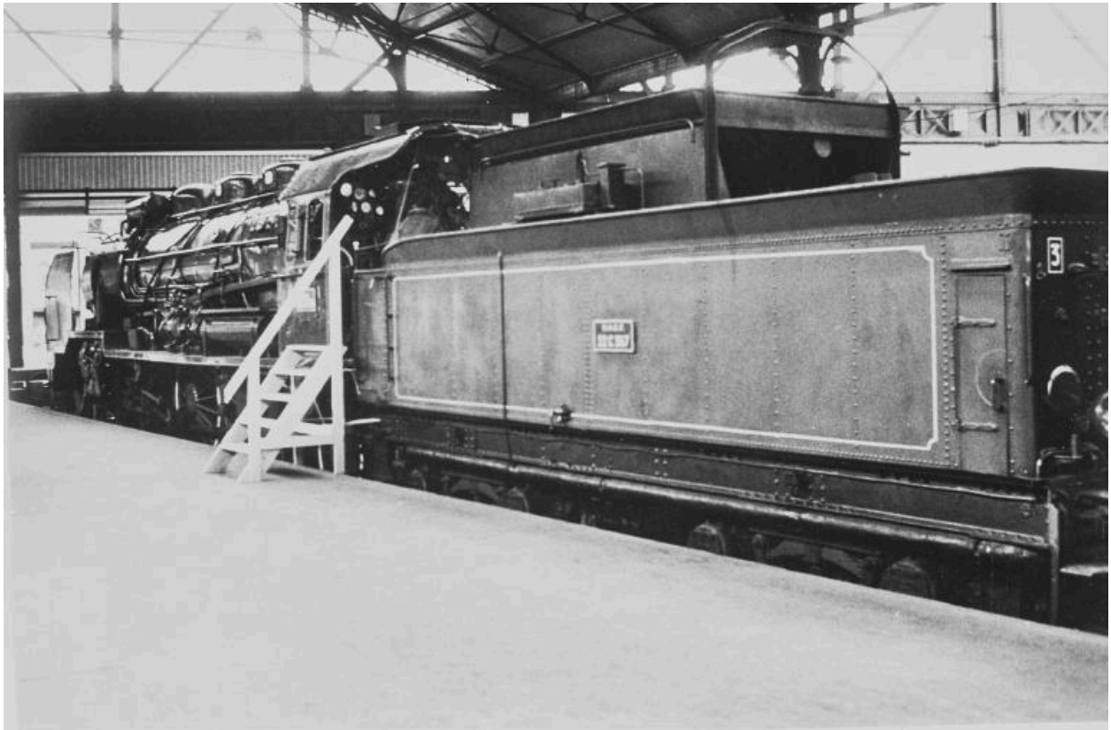
Locomotive et tender, vue latérale gauche, pendant les travaux de restauration.- Photographie, vers 1985 (Coll. part.).
