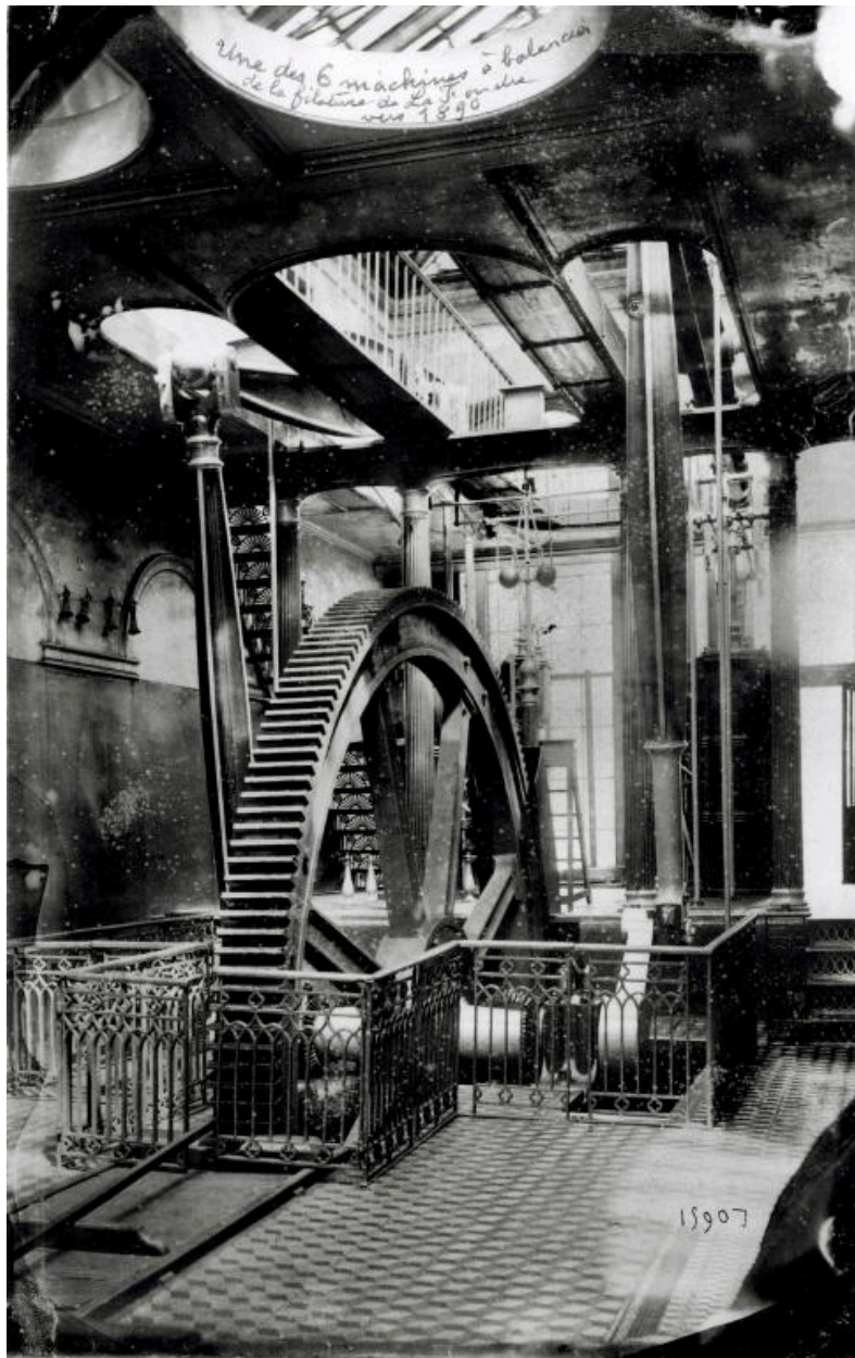
Vue intérieure de la salle des machines à vapeur, détail d'une des 6 machines à balancier de la filature la Foudre.- Photographie, vers 1890 (AM, Petit-Quevilly).
