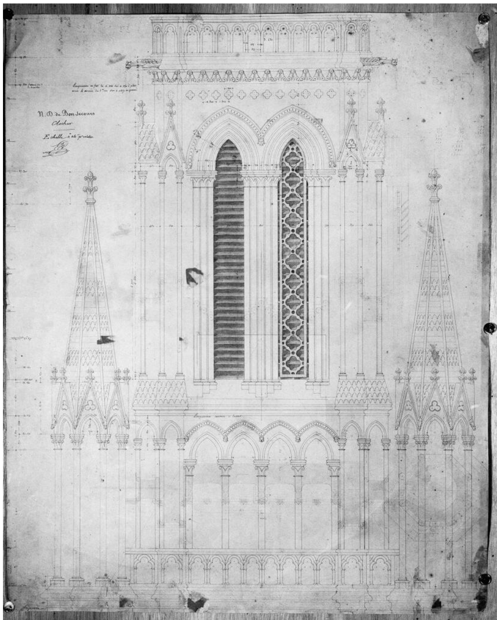
Base du clocher, élévation.- Dessin, Barthélémy architecte, sans date, [vers 1840]. (Archives diocésaines de Rouen).
