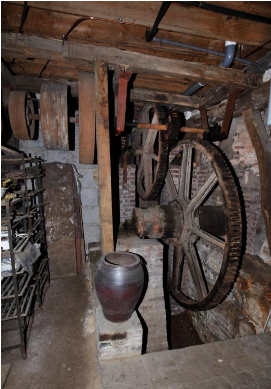
Vue intérieure du moulin : engrenages et arbre de transmission.
