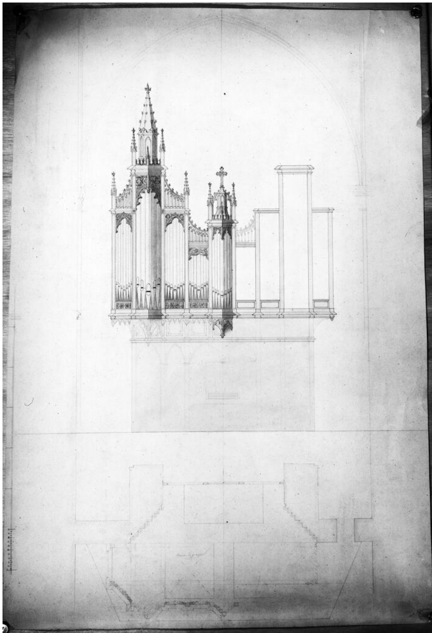
Buffet d'orgue.- Dessin, Barthélémy architecte, sans date, [vers 1860]. (Archives diocésaines de Rouen).
