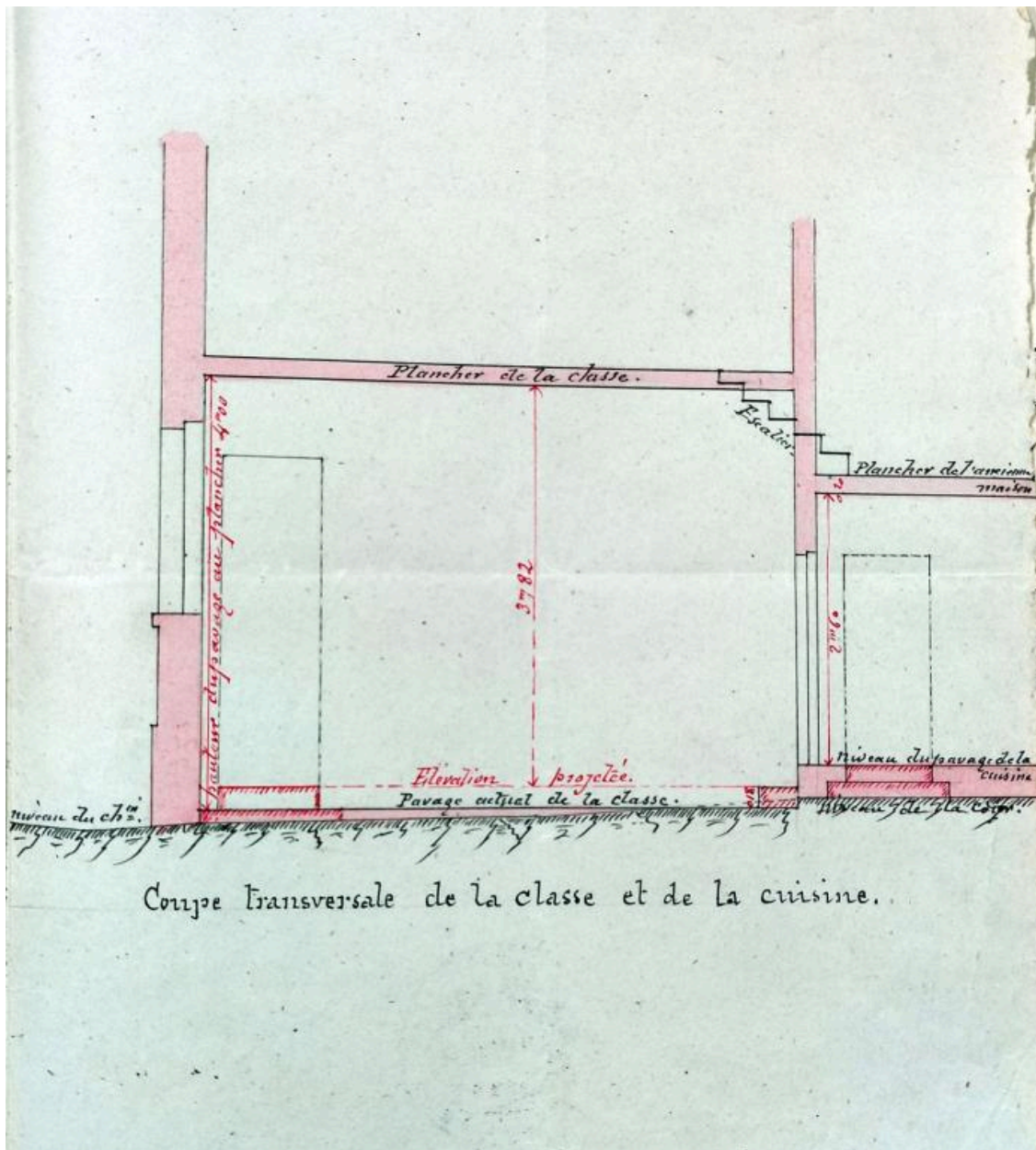
Coupe transversale de la classe et de la cuisine, 1866.
