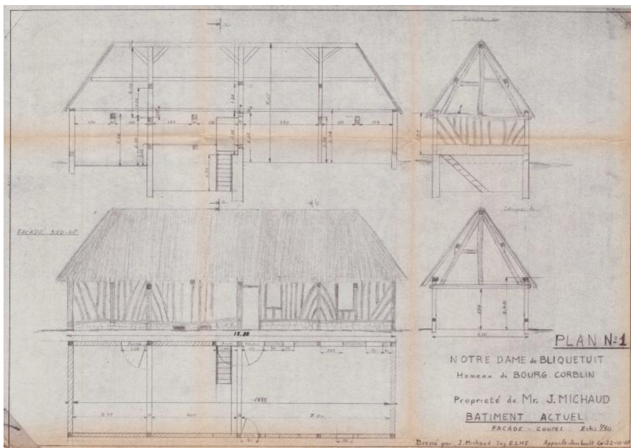
Plan et coupes du bâtiment d'origine dressé par Jean Michaud, 22 octobre 1967.
