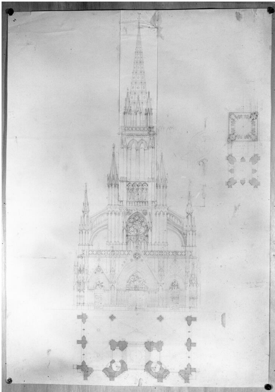
Façade occidentale, élévation et plan.- Dessin, Barthélémy architecte, sans date, [vers 1850]. (Archives diocésaines de Rouen).
