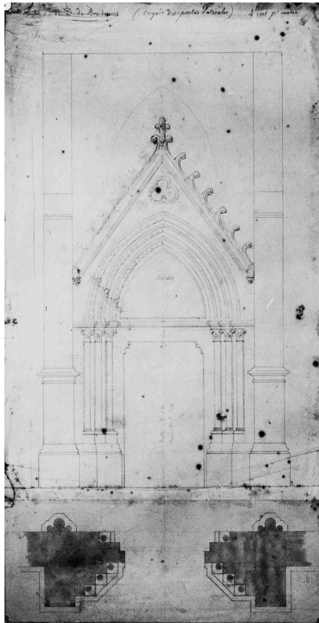
Portes latérales, croquis (élévation - plan).- Dessin, plan n° 97, Barthélémy architecte, sans date, [vers 1840]. (Archives diocésaines de Rouen).
