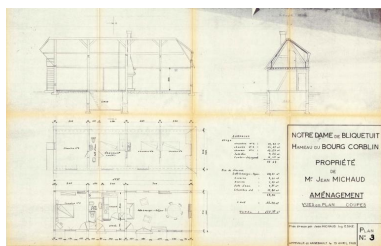
Plan et coupes de l'aménagement intérieur dressé par M. Michaud, 15 avril 1968. Repro. Gaëlle Pottier IVR28_20197606268NUCA
