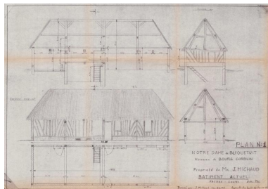
Plan et coupes du bâtiment d'origine dressé par Jean Michaud, 22 octobre 1967. Repro. Gaëlle Pottier IVR28_20197606266NUCA
