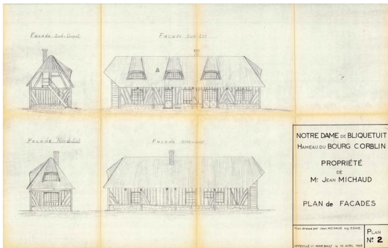
Plan de façades dressé par M. Michaud, 15 avril 1968.
