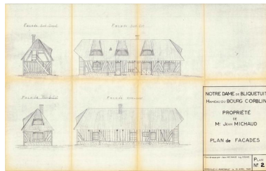
Plan de façades dressé par M. Michaud, 15 avril 1968. Repro. Gaëlle Pottier IVR28_20197606267NUCA
