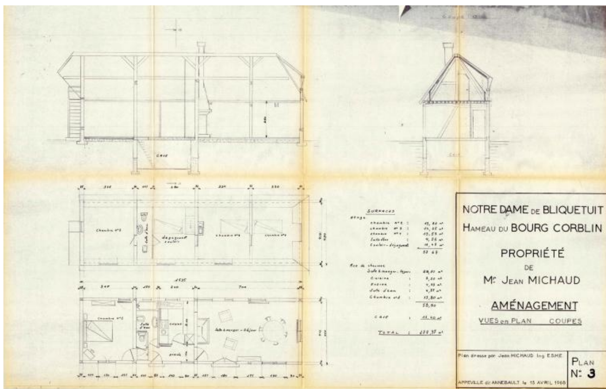
Plan et coupes de l'aménagement intérieur dressé par M. Michaud, 15 avril 1968.
